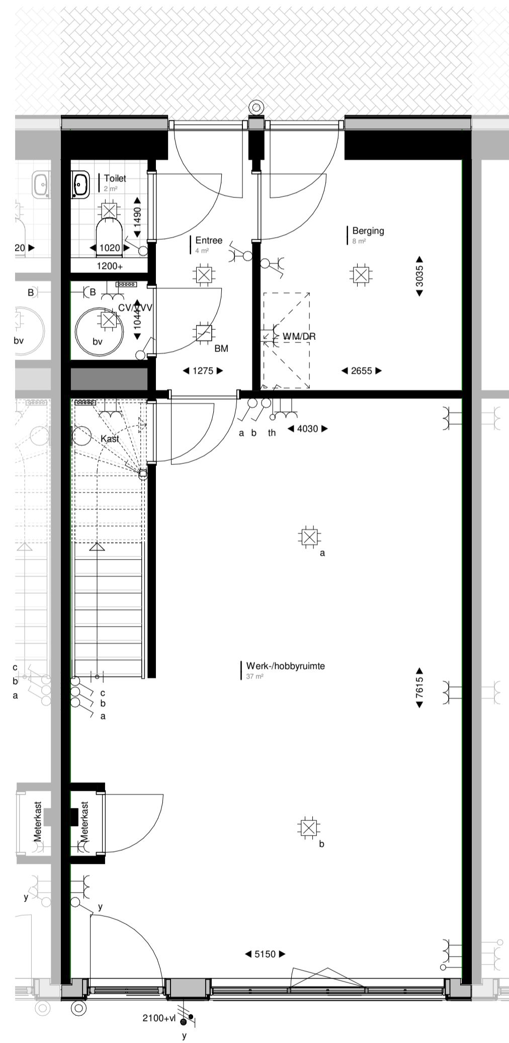
Begane grond 1:50
