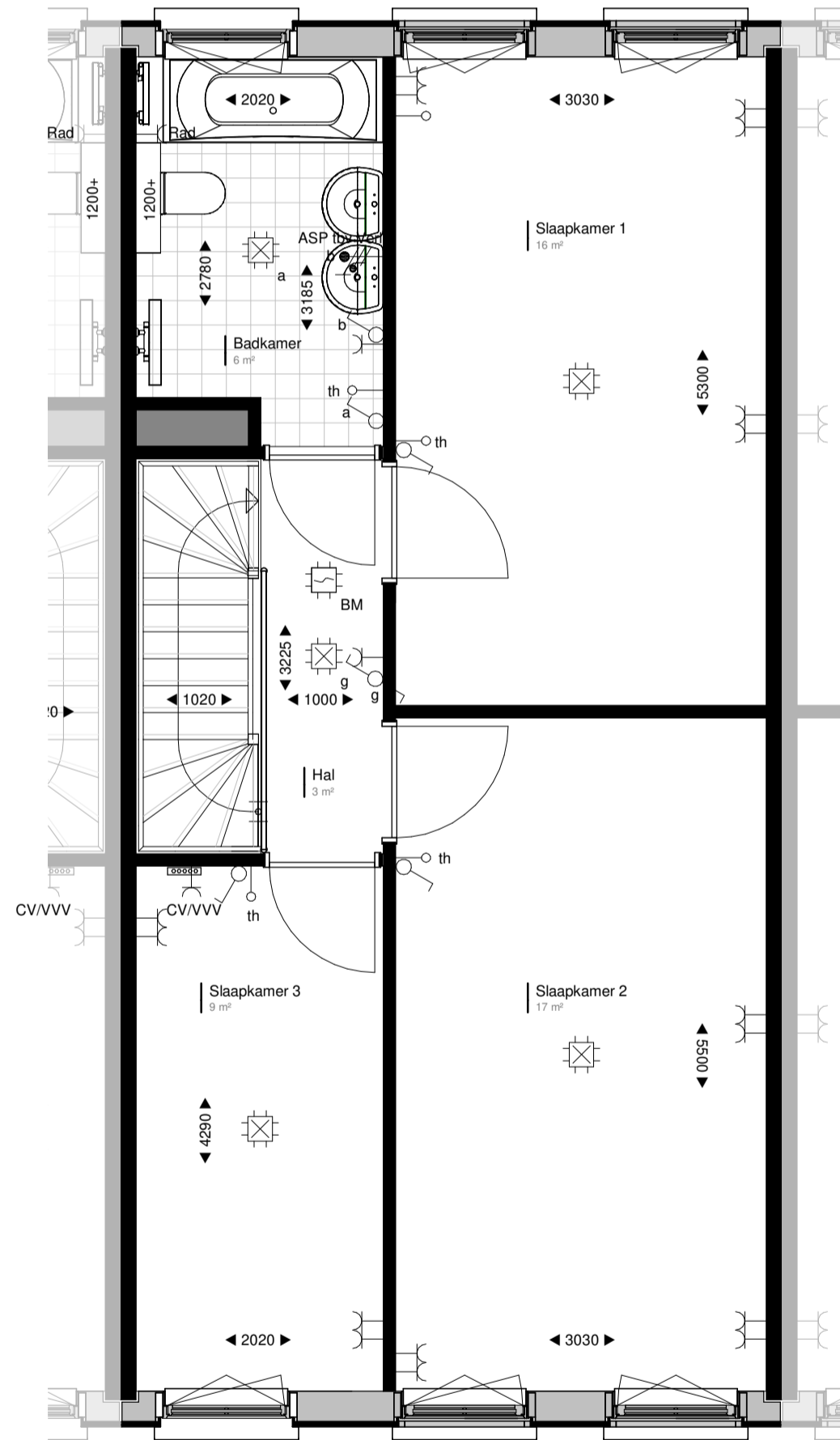
Tweede verdieping 1:50
