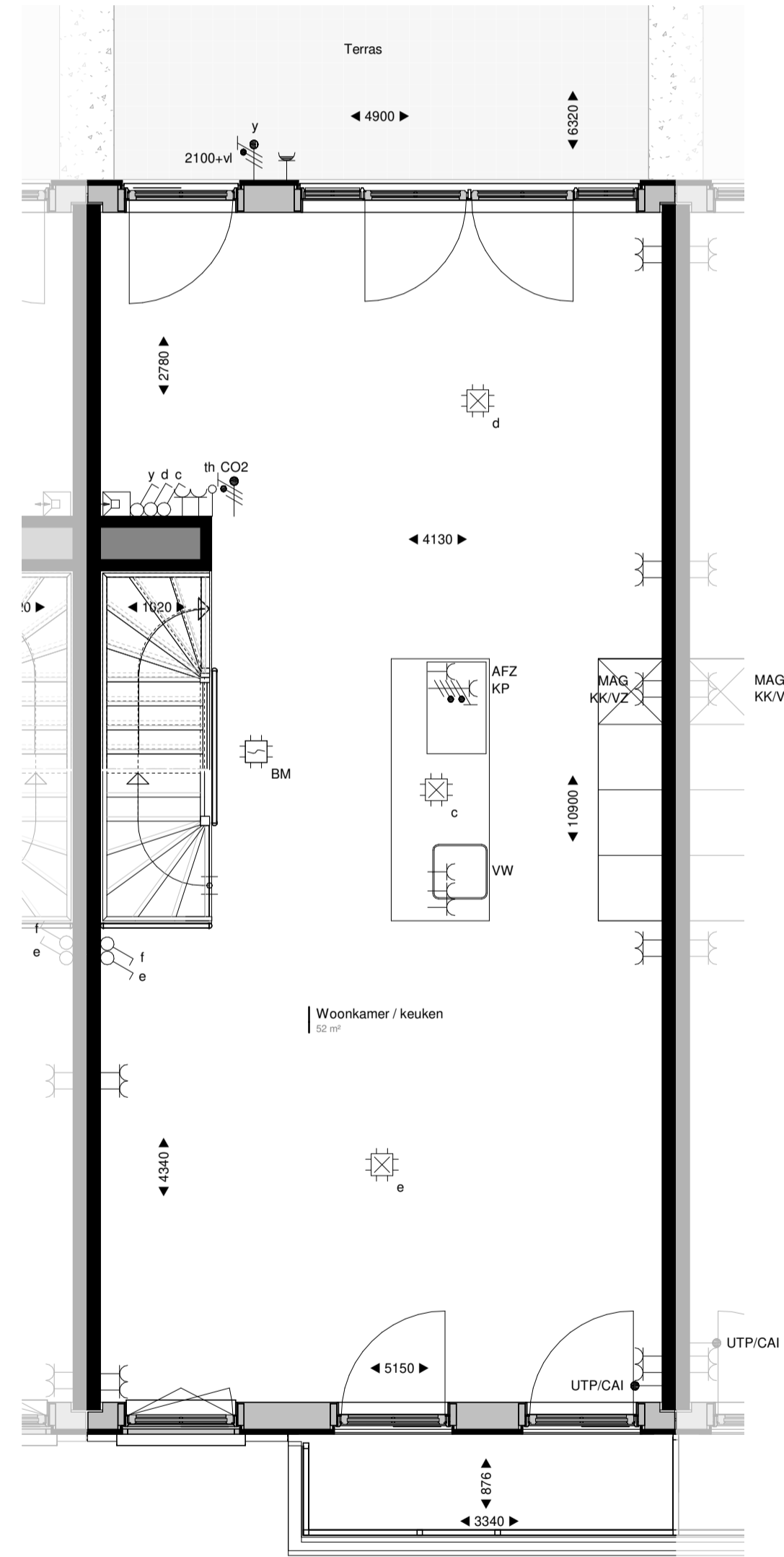
Eerste verdieping 1:50
