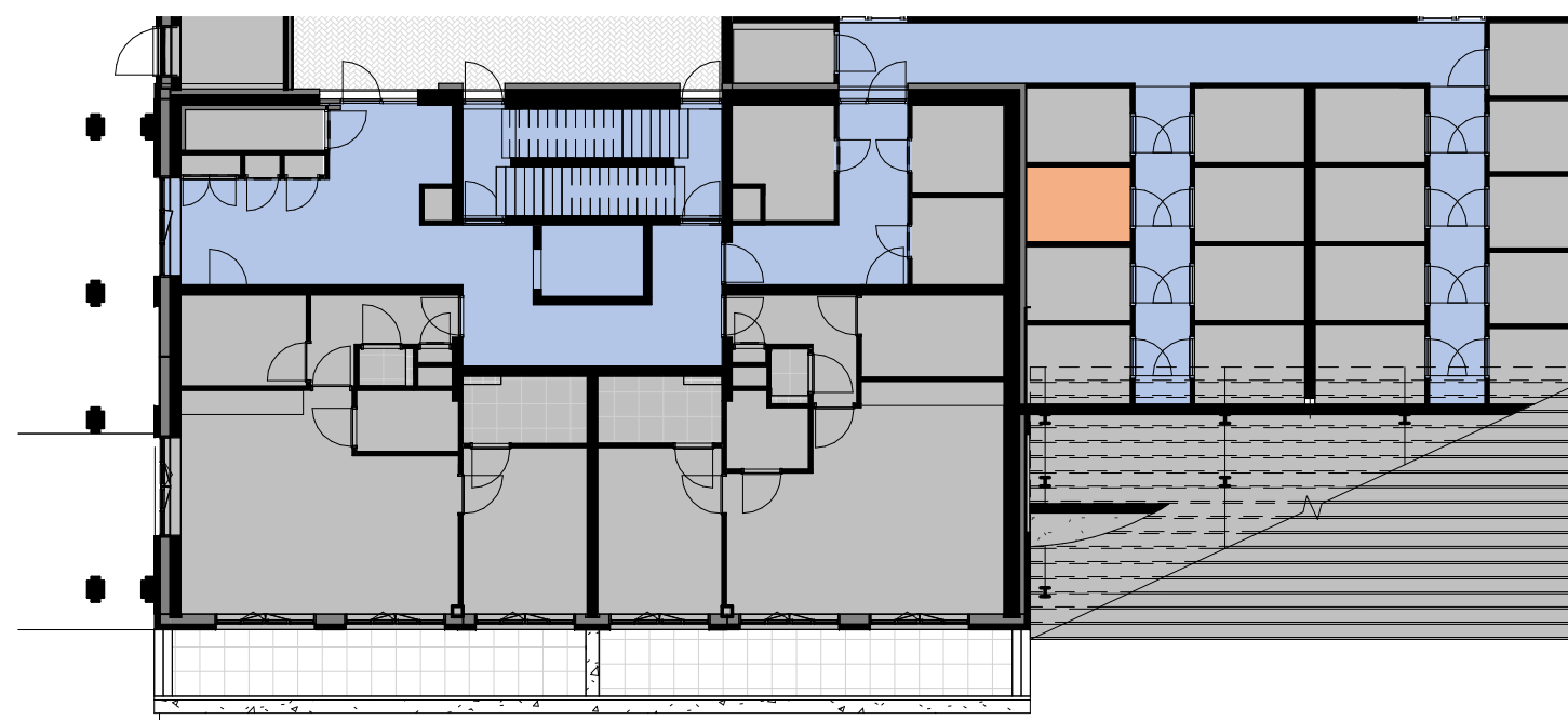
Bergring aanduiding 1 : 200
