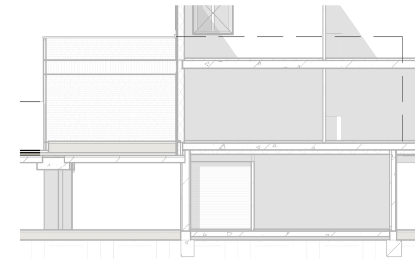
Linker zijgevel 1:200
