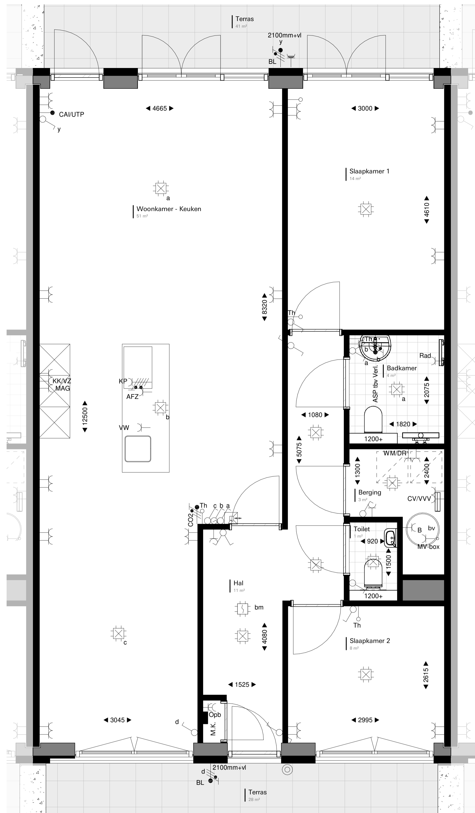
Verdieping 1 1:50
