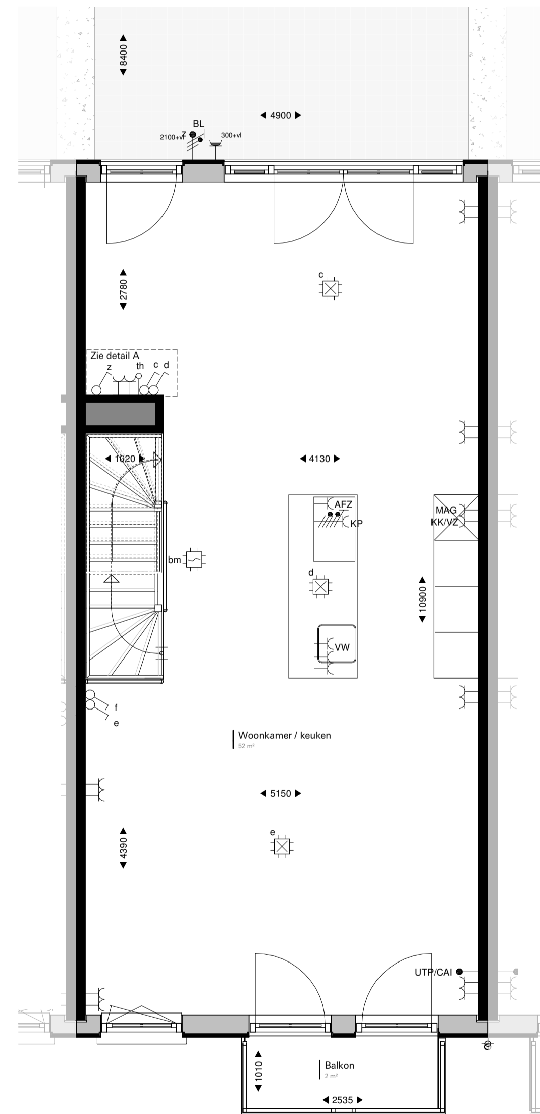
Verdieping 1 1:50
