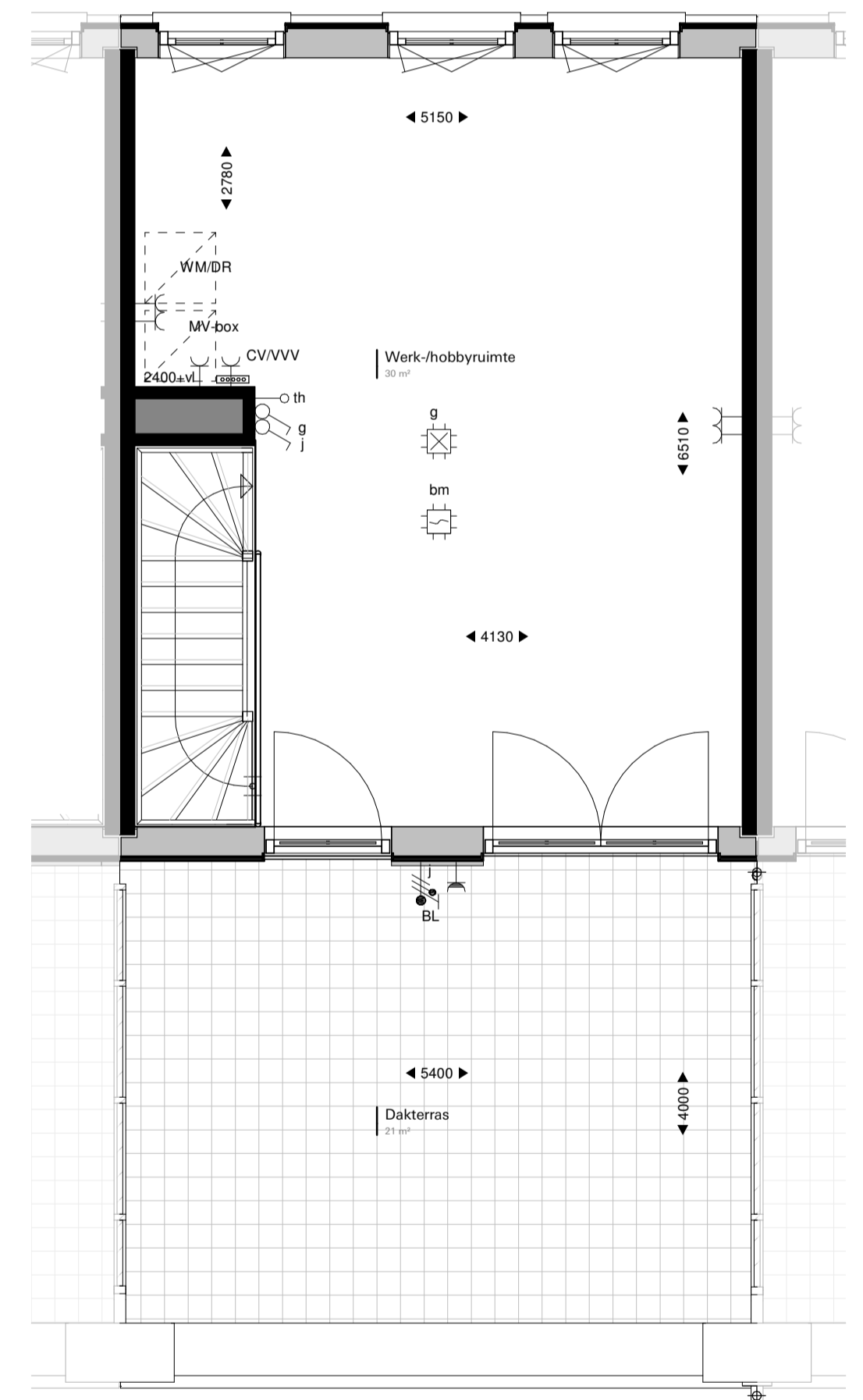
Verdieping 3 1:50
