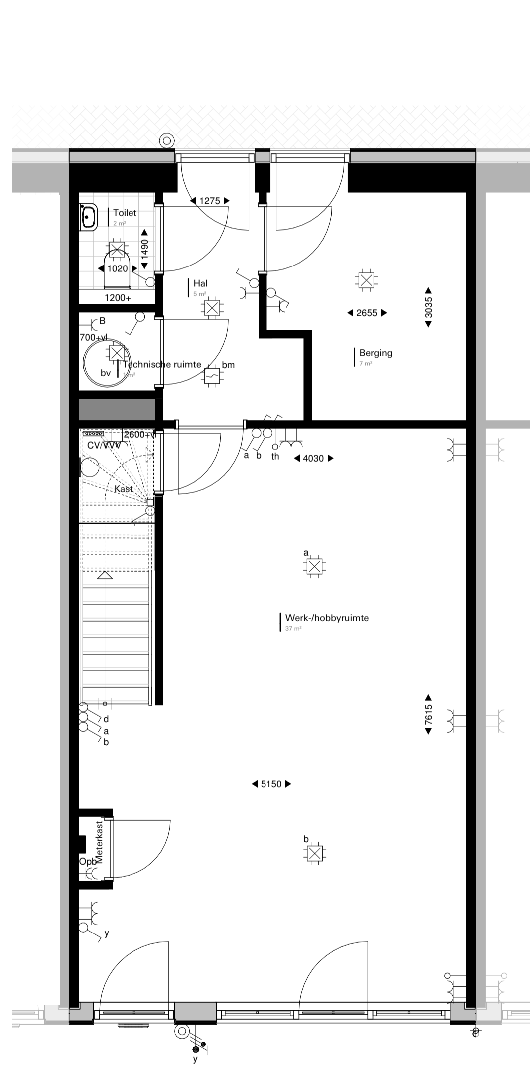
Begane grond 1:50
