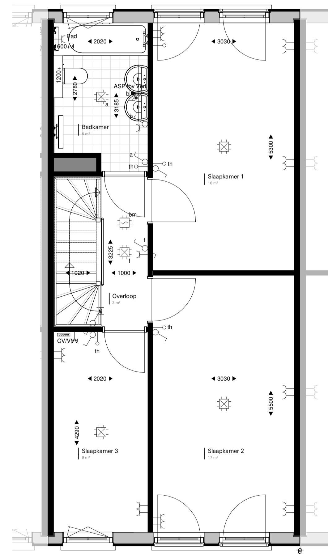
Verdieping 2 1:50
