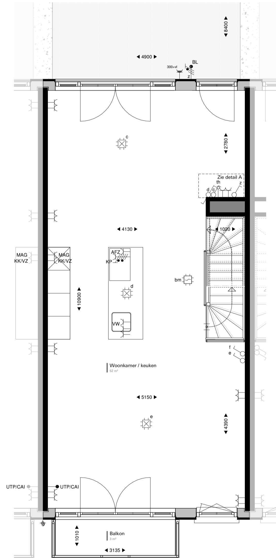
Verdieping 1 1:50
