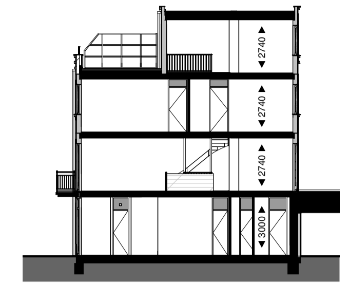
Doorsnede 1:200
