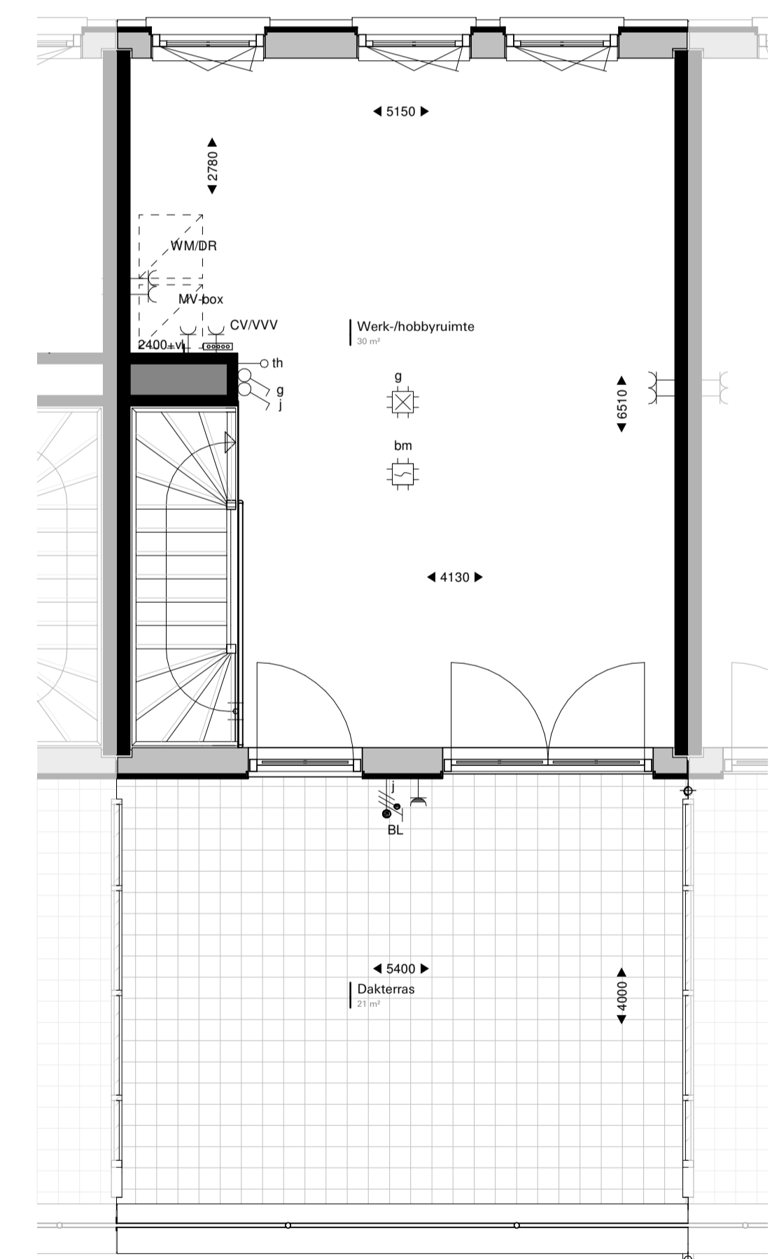
Verdieping 3 1:50
