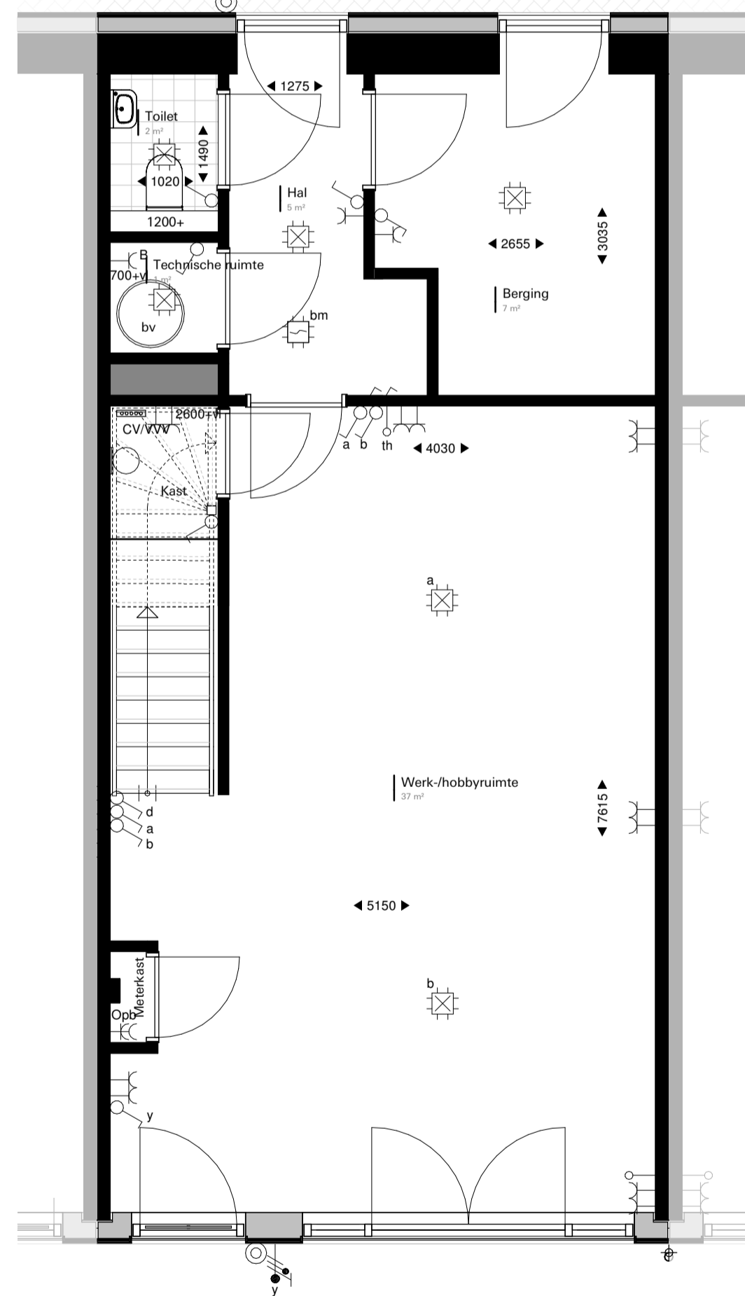
Begane grond 1:50
