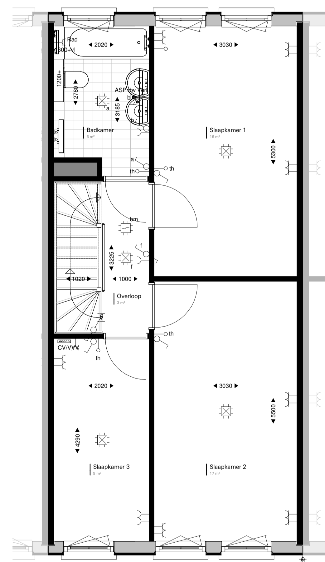
Verdieping 2 1:50
