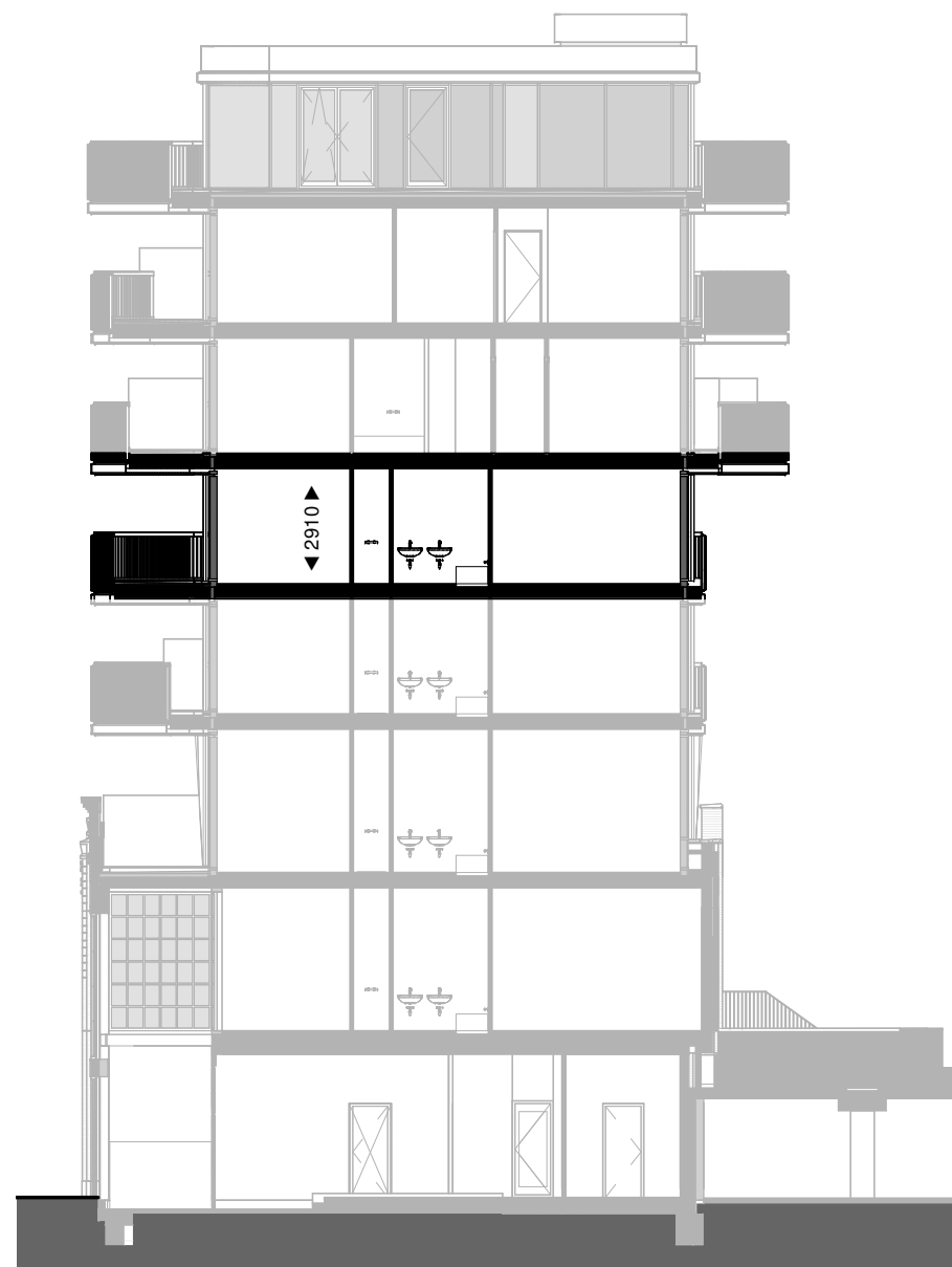
VK.E.17_doorsnede 1 : 200
