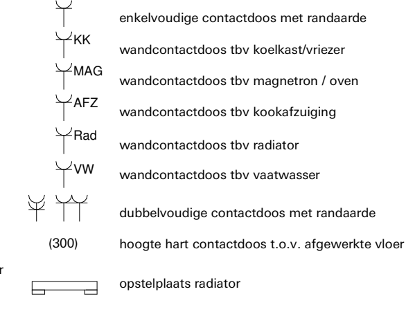
Berging Aanduiding 1 : 200
