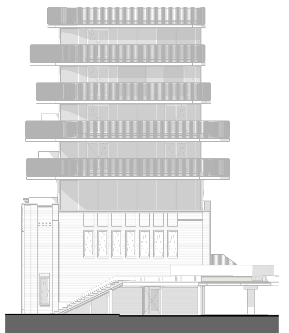
VK.E.17_Rechter zijgevel 1 : 200
