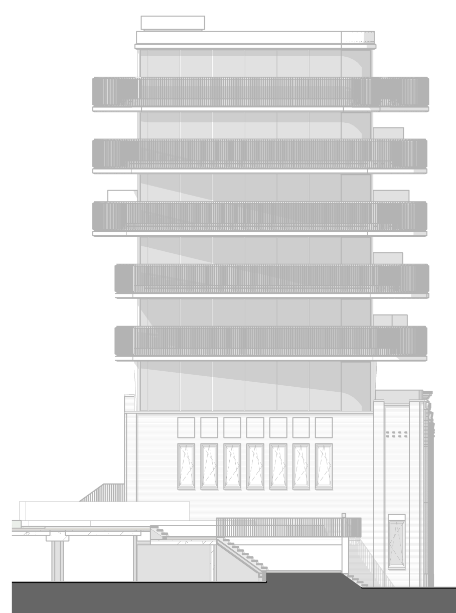
VK.E.17_Linker zijgevel 1 : 200
