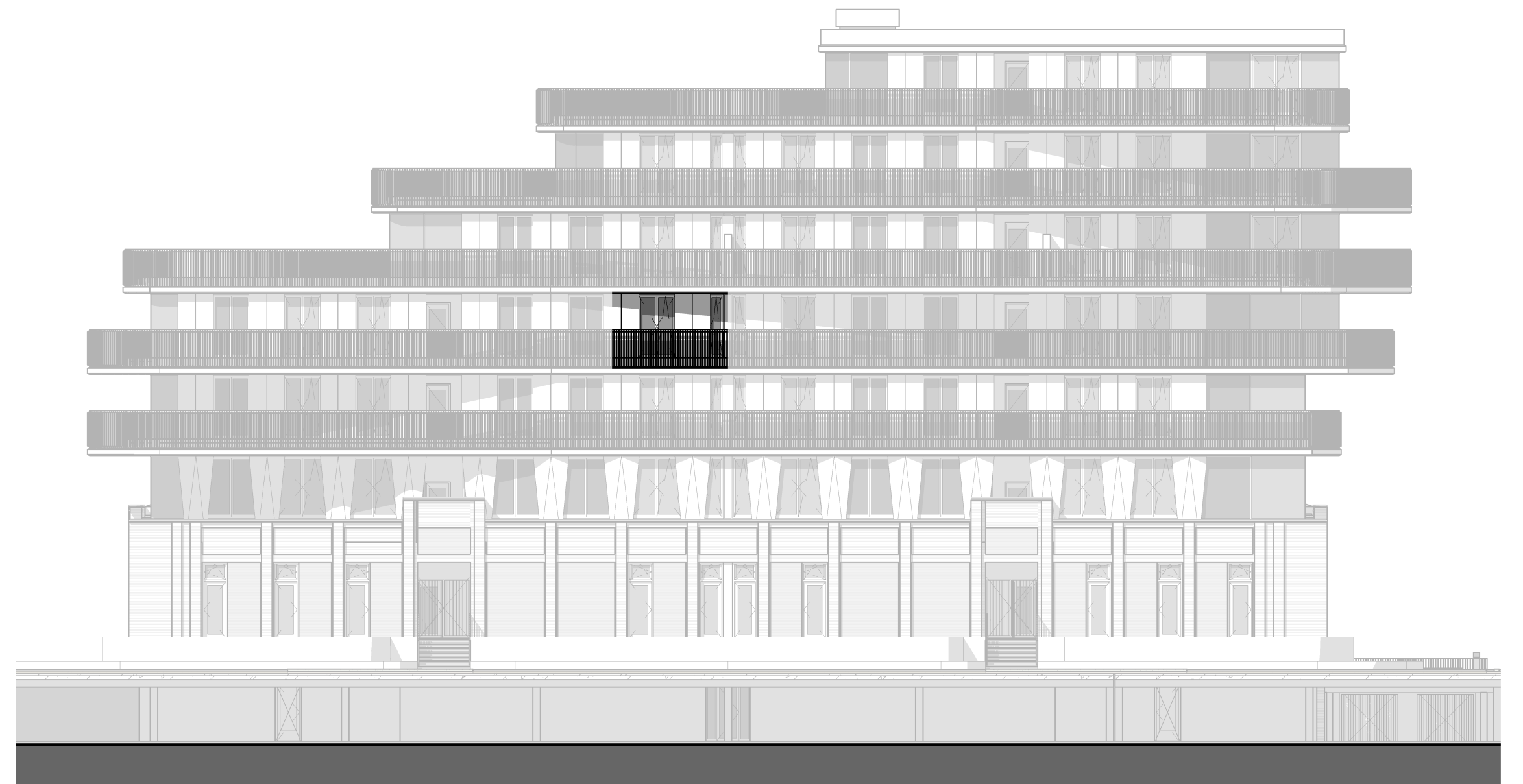
VK.E.17_Achtergevel 1 : 200
